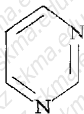
Пиримидин (1,3-диазин)
