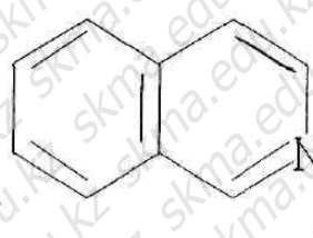
изохинолин
