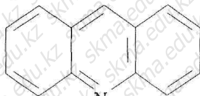
Акридин
