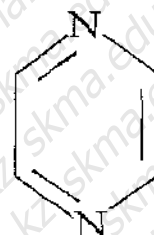
Пиазин (1,4-диазин)
